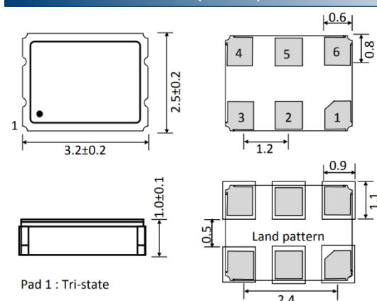
Dimensions(Unit:mm)
