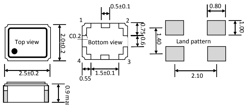
Dimensions(Unit:mm)
