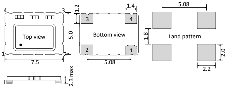
Dimensions (Unit:mm)
